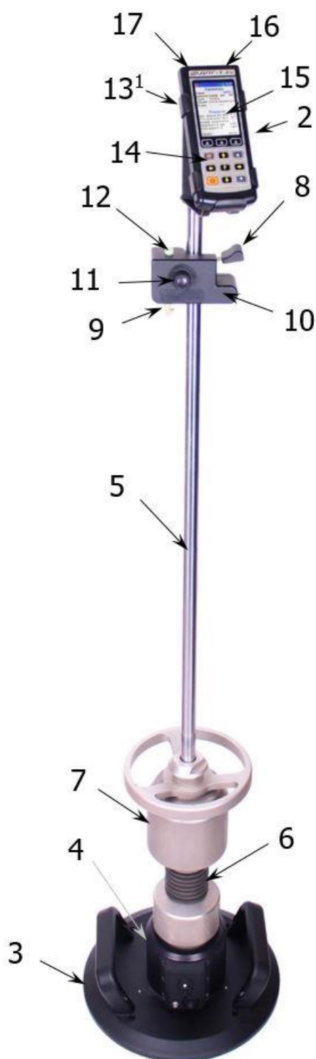
Рисунок 1 – Общий вид прибора ДПГ-1.2
